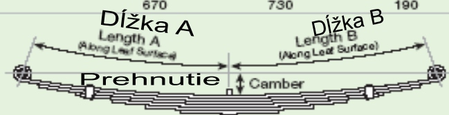
Jedno stupňová pružina
