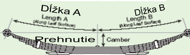
Dvoj stupňová pružina
