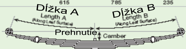
Jedno stupňová pružina
